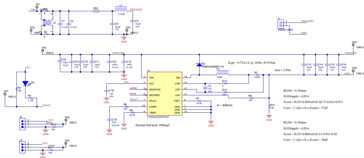
図 3-1. LP8868ZQ1EVM の回路図
