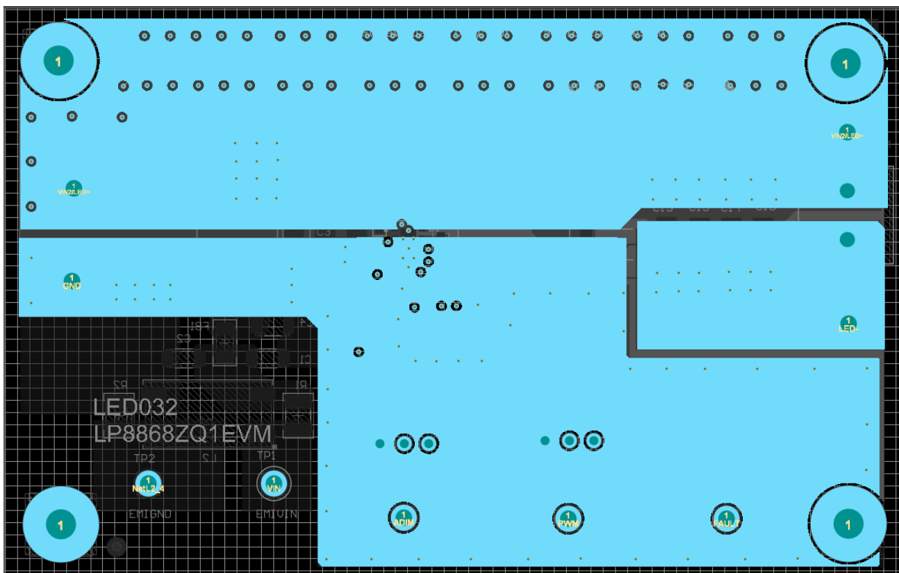
図 3-4. LP8868ZQ1EVM 内層 2
