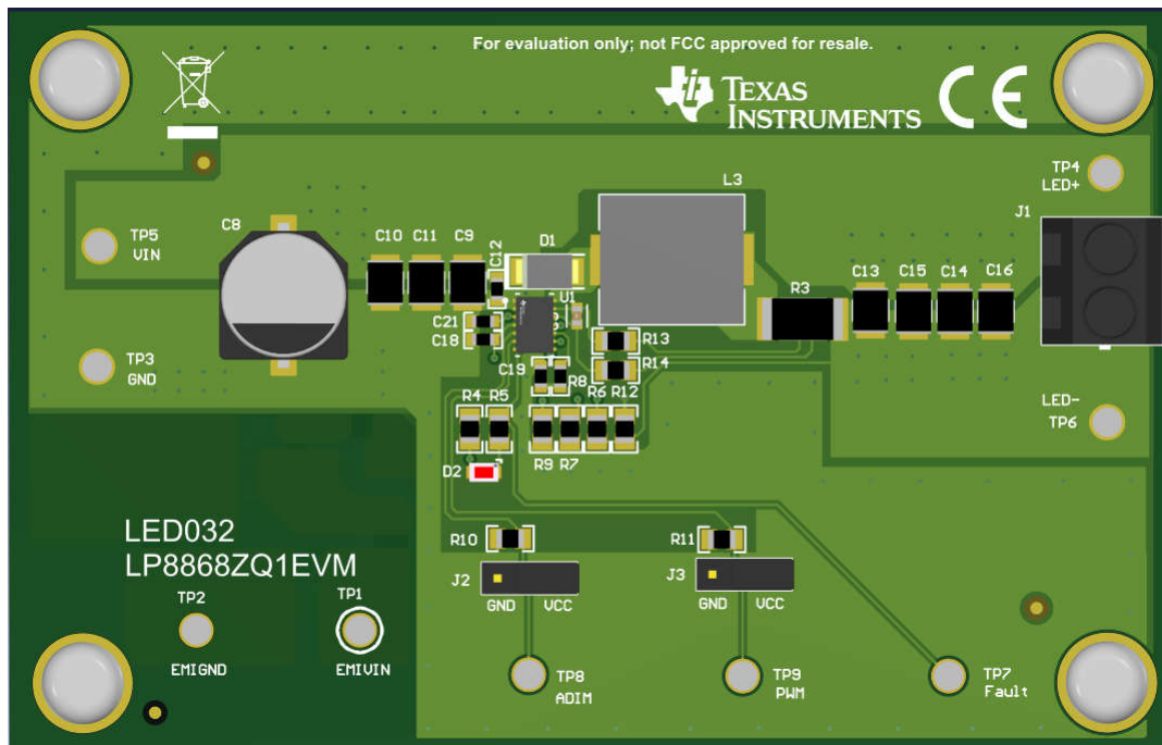
図 1-1. LP8868ZQ1EVM キット
