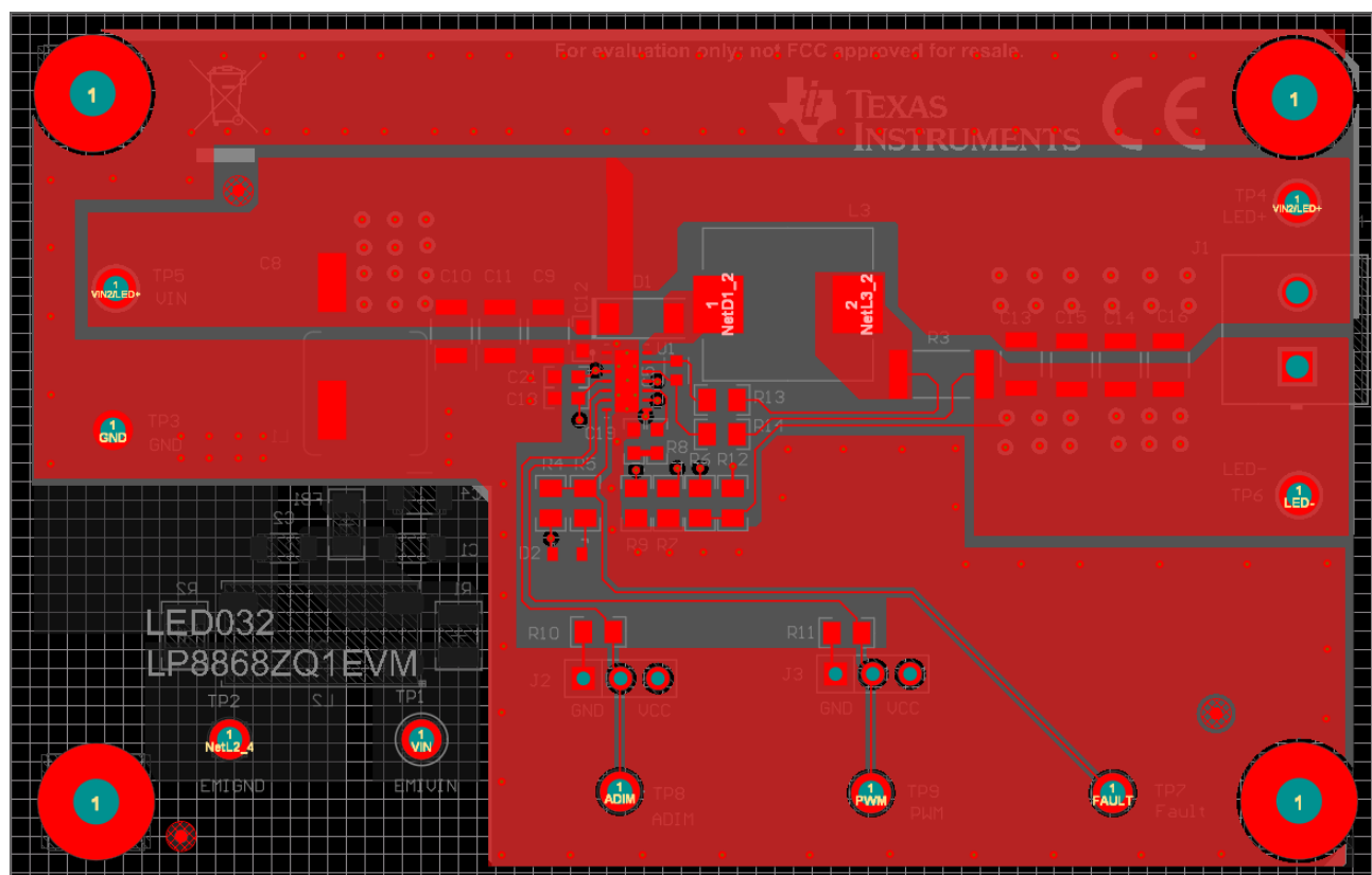
図 3-2. LP8868ZQ1EVM 最上層
