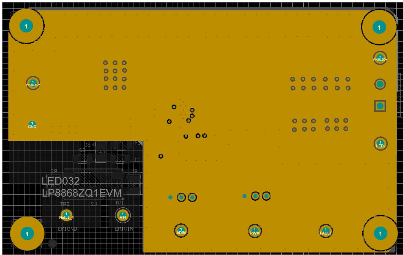
図 3-3. LP8868ZQ1EVM 内層 1
