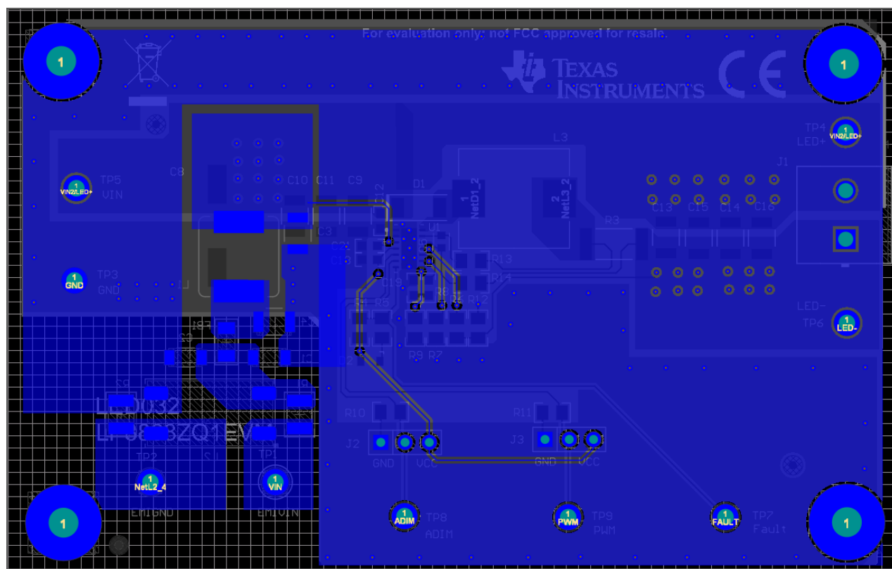
図 3-5. LP8868ZQ1EVM 最下層
