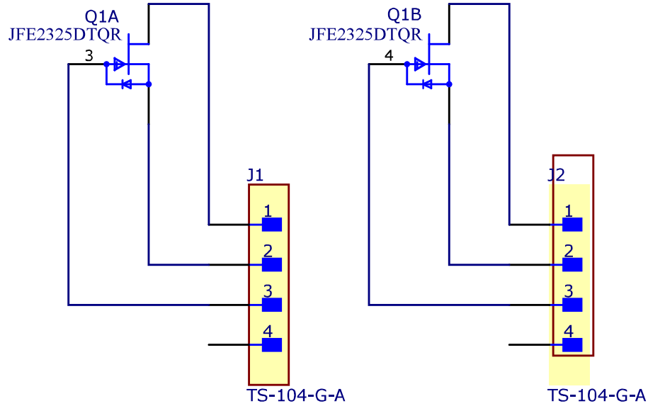
図 3-1. JFE2325EVM の回路図
