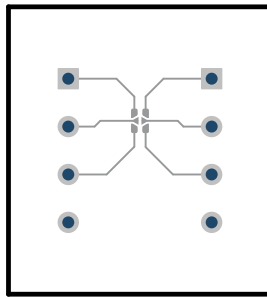
図 3-4. JFE2325EVM PCB 最上層
