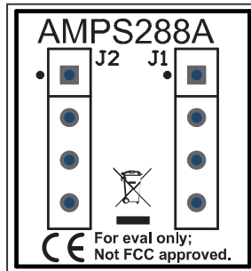
図 3-5. JFE2325EVM PCB コンポジット (底面図)
