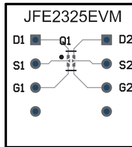
図 3-2. JFE2325EVM PCB レイアウト コンポジット (上面図)
