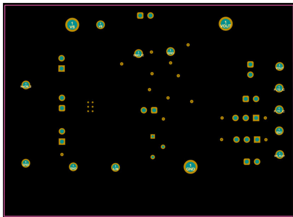
図 4-3. TPS1HC120Q1EVM の第 2 層
