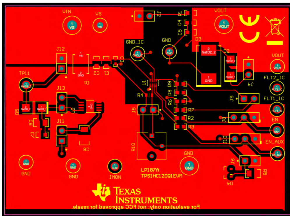
図 4-2. TPS1HC120Q1EVM 最上層
