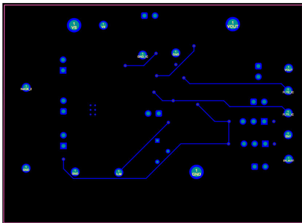
图 4-5. TPS1HC120Q1EVM 最下層
