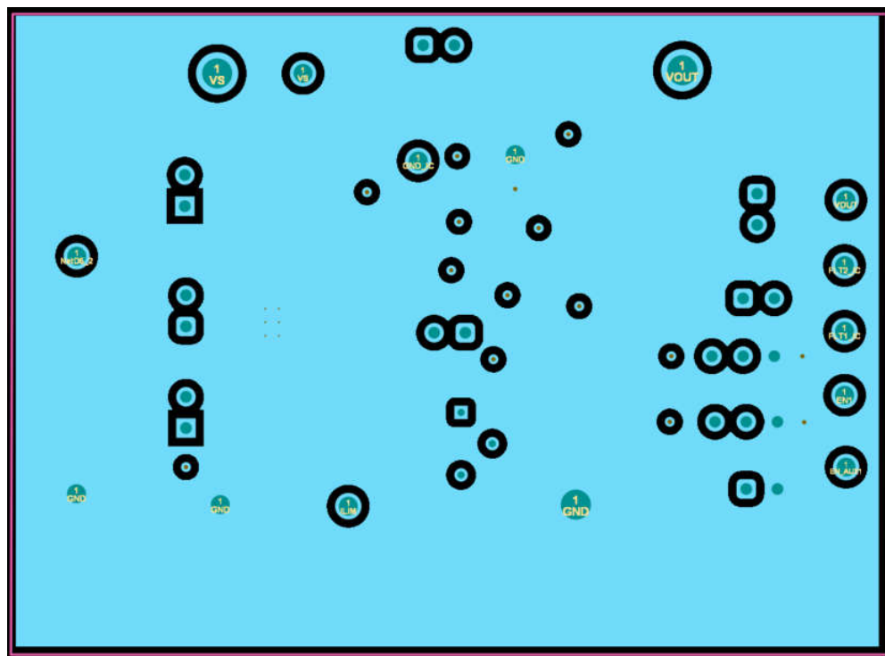
図 4-4. TPS1HC120Q1EVM の第 3 層 (グランド)
