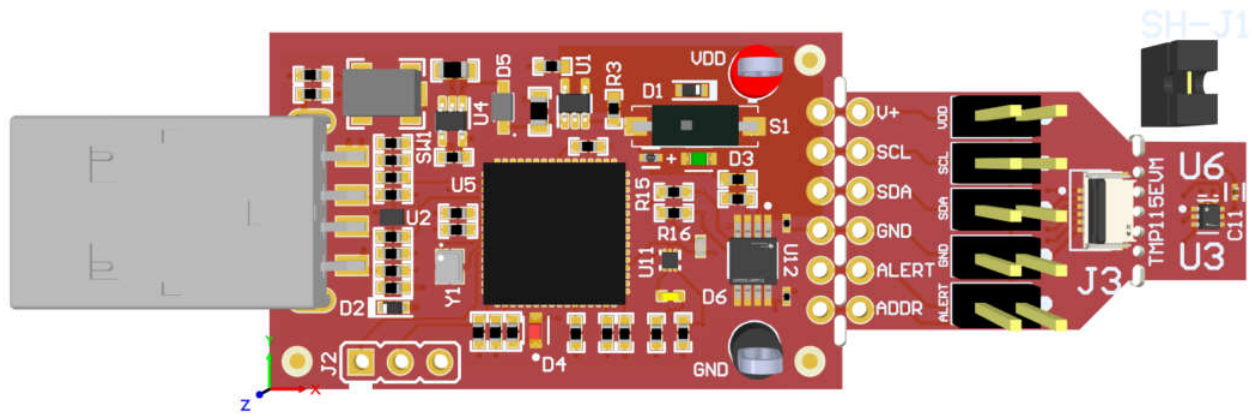
TMP115EVM
