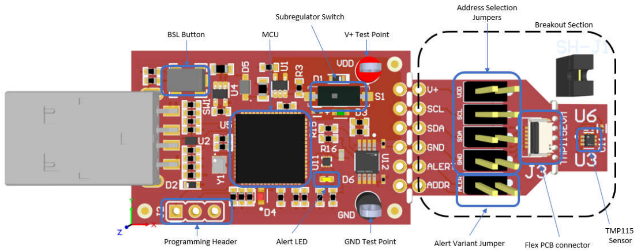
図 2-1. TMP115EVM 基板セクション
