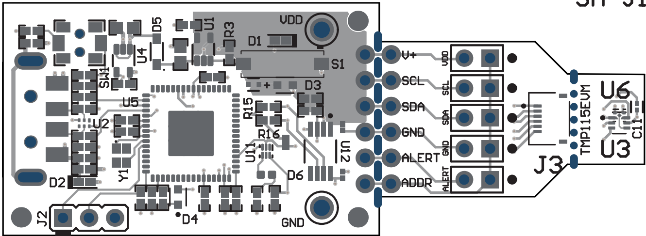
図 4-2. 上面図
