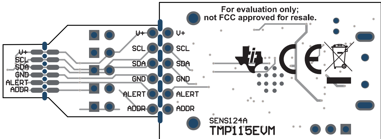
図 4-3. 底面図
