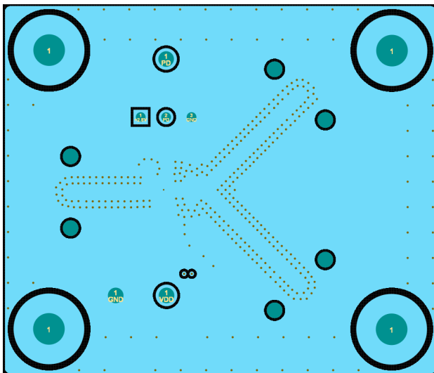
図 3-4. 第3層
