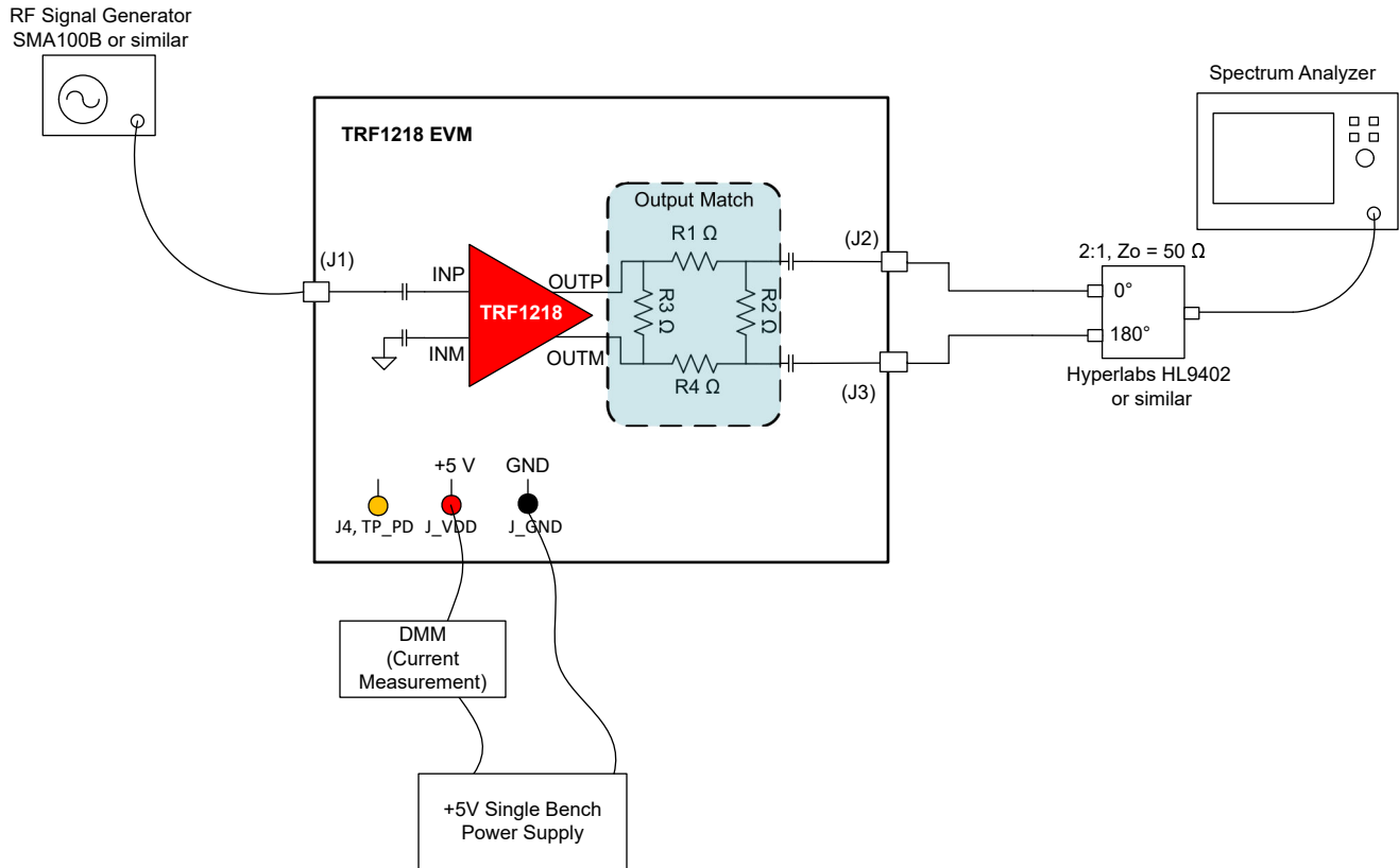
図 2-1. ゲインおよび OP1dB のテスト構成
