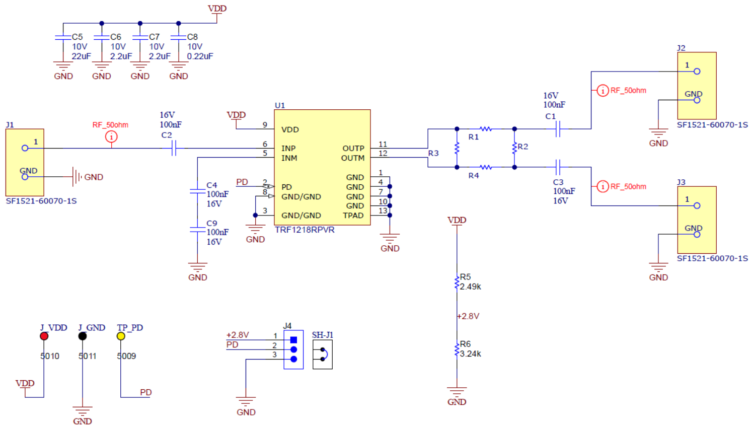
図 3-1. TRF1218EVM の回路図
