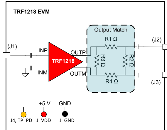
図 1-1. TRF1218EVM の機能ブロック図
