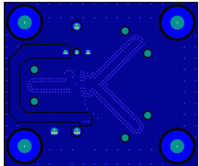
図 3-5. 下層
