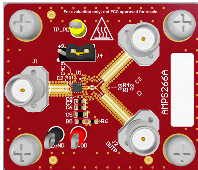
TRF1218EVM
