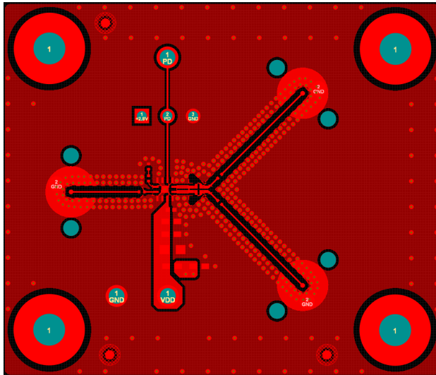
図 3-2. 上層
