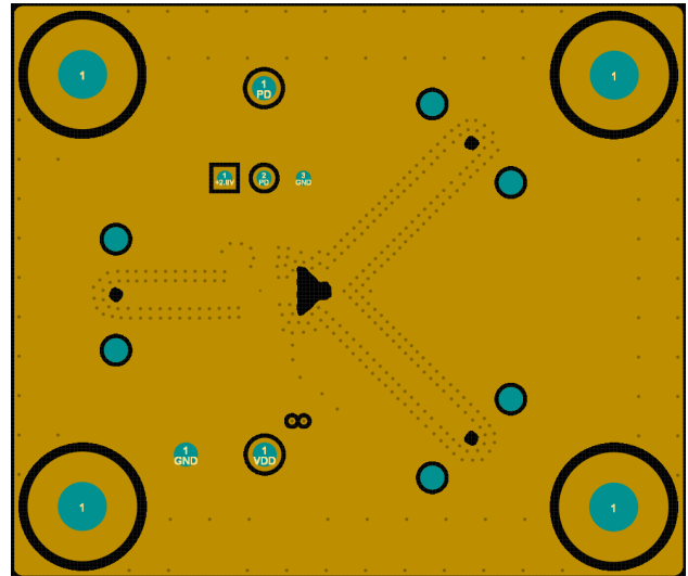
図 3-3. 第2層
