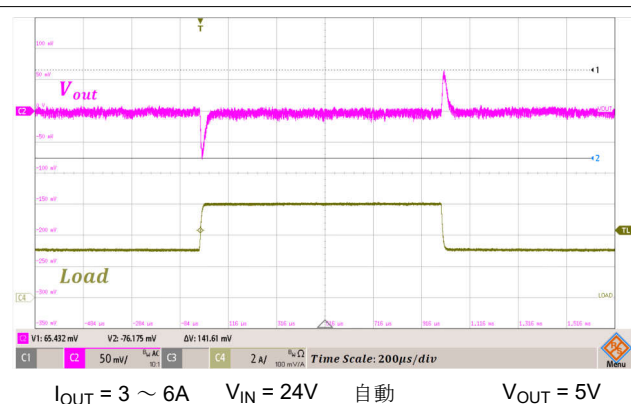
図 3-8. 負荷過渡
