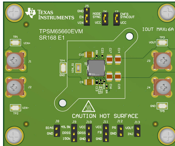
図 2-1. TPSM65660EVM の上面
