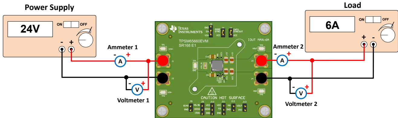
図 2-3. TPSM65660EVM の設定
