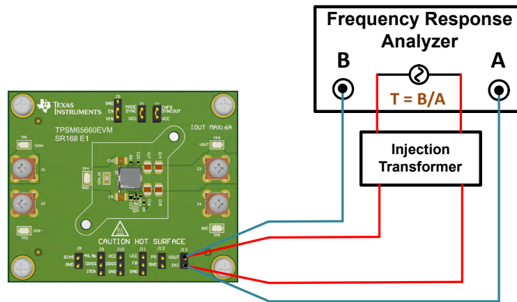
図 2-4. TPSM65660EVM ボード接続
