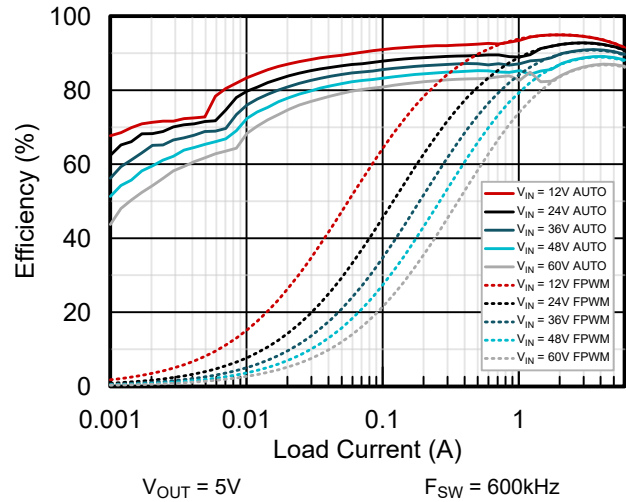
図 3-2. 効率
