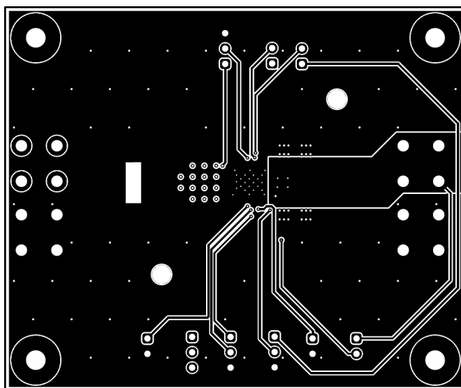
図 4-5. PCB 信号レイヤ 2
