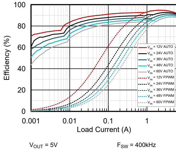
図 3-1. 効率
