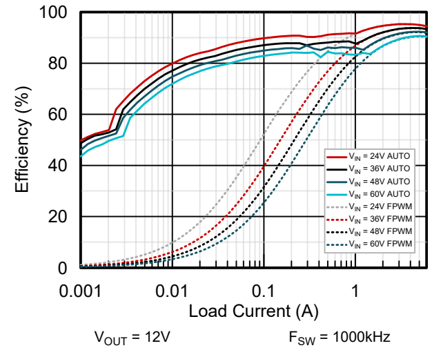
図 3-4. 効率
