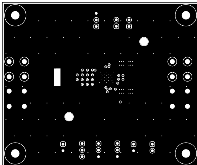
図 4-4. PCB 信号レイヤ 1
