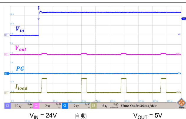
図 3-6. 出力短絡での起動
