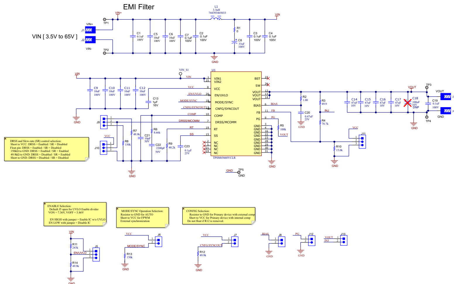
図 4-1. TPSM65660EVM の回路図
