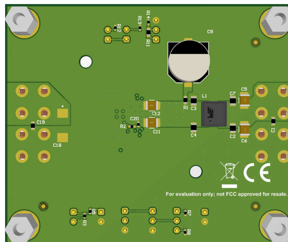
図 2-2. TPSM65660EVM 底面
