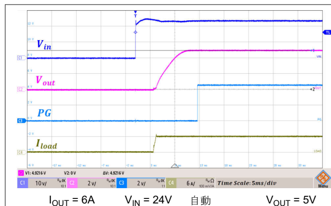
図 3-5. 全負荷での起動
