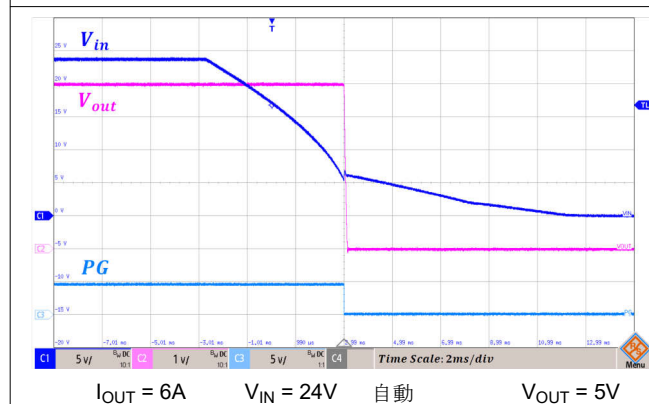
図 3-7. シャットダウン
