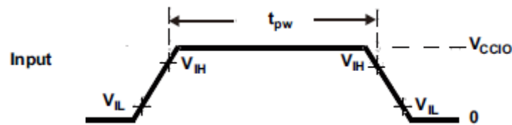
図 3-2 TTL レベル入力
