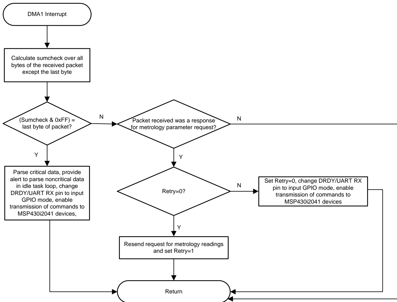
図 14. DMA1 ISR
