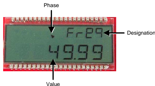
図 29. LCD
