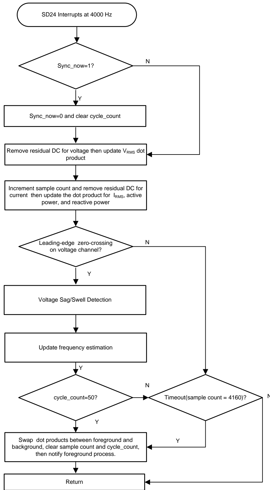
図 10. per_sample_dsp Function
