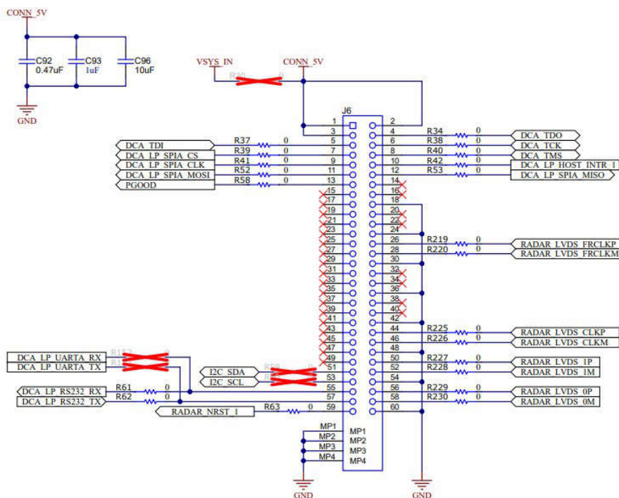
図 3-16. DCA1000 HD コネクタ ピン
