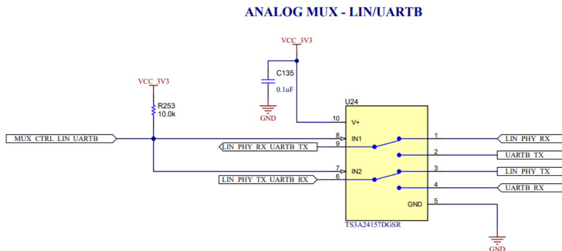
図 3-25. LIN PHY スイッチ用アナログ マルチプレクサ
