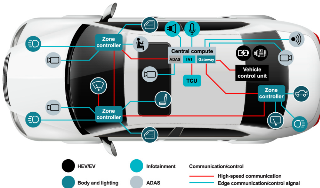
圖 2. 軟體定義車輛中中央運算架構與連網系統簡化概覽
