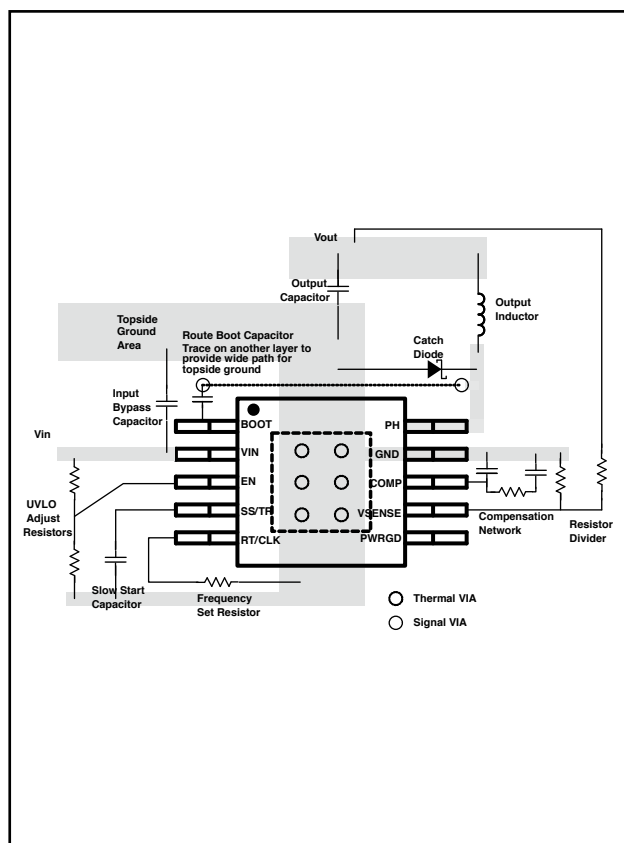
PCBレイアウト例
