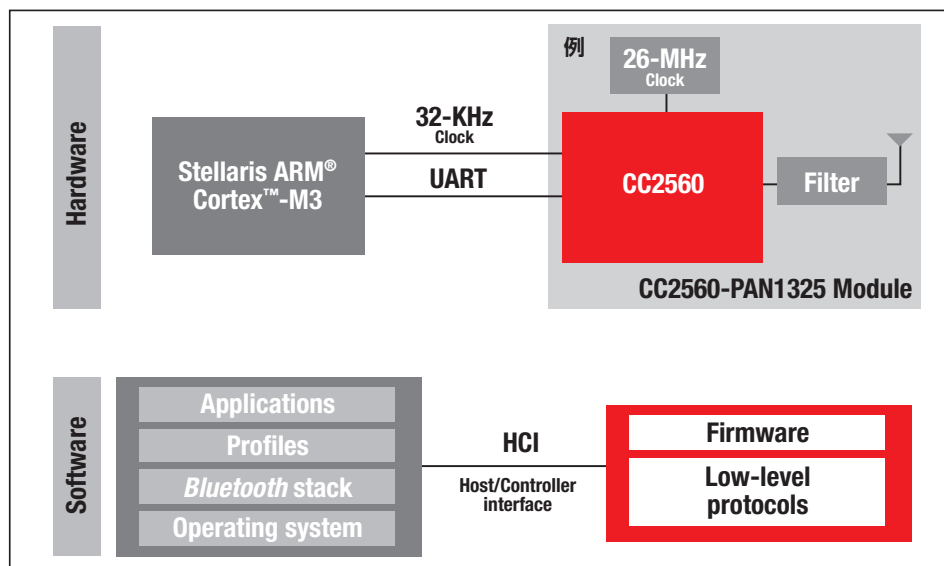
▲ CC2560-PAN1325 Bluetooth システム
