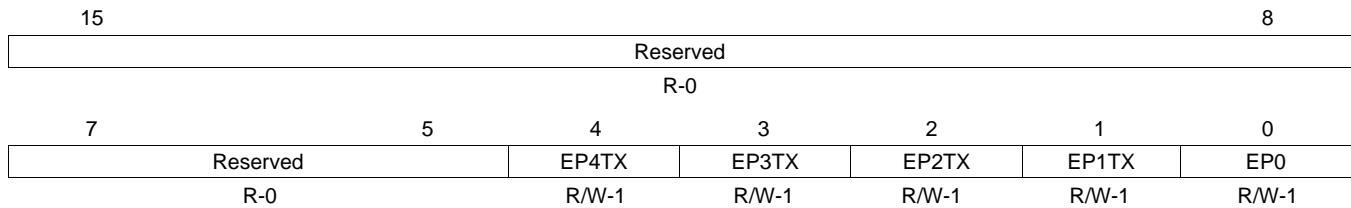
Figure 51. Interrupt Enable Register for INTRTX (INTRTXE)
