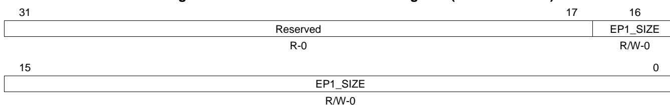
Figure 43. Generic RNDIS EP1 Size Register (GENRNDISSZ1)
