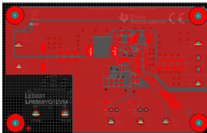
Figure 3-2. LP8868YQ1EVM Top Layer
