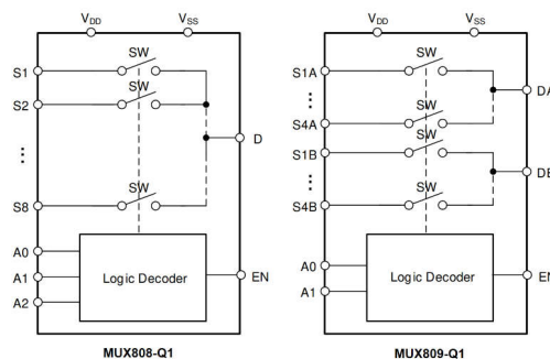
MUX808-Q1 and MUX809-Q1 Block Diagram
