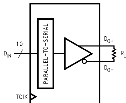
Figure 18. V OD Diagram
