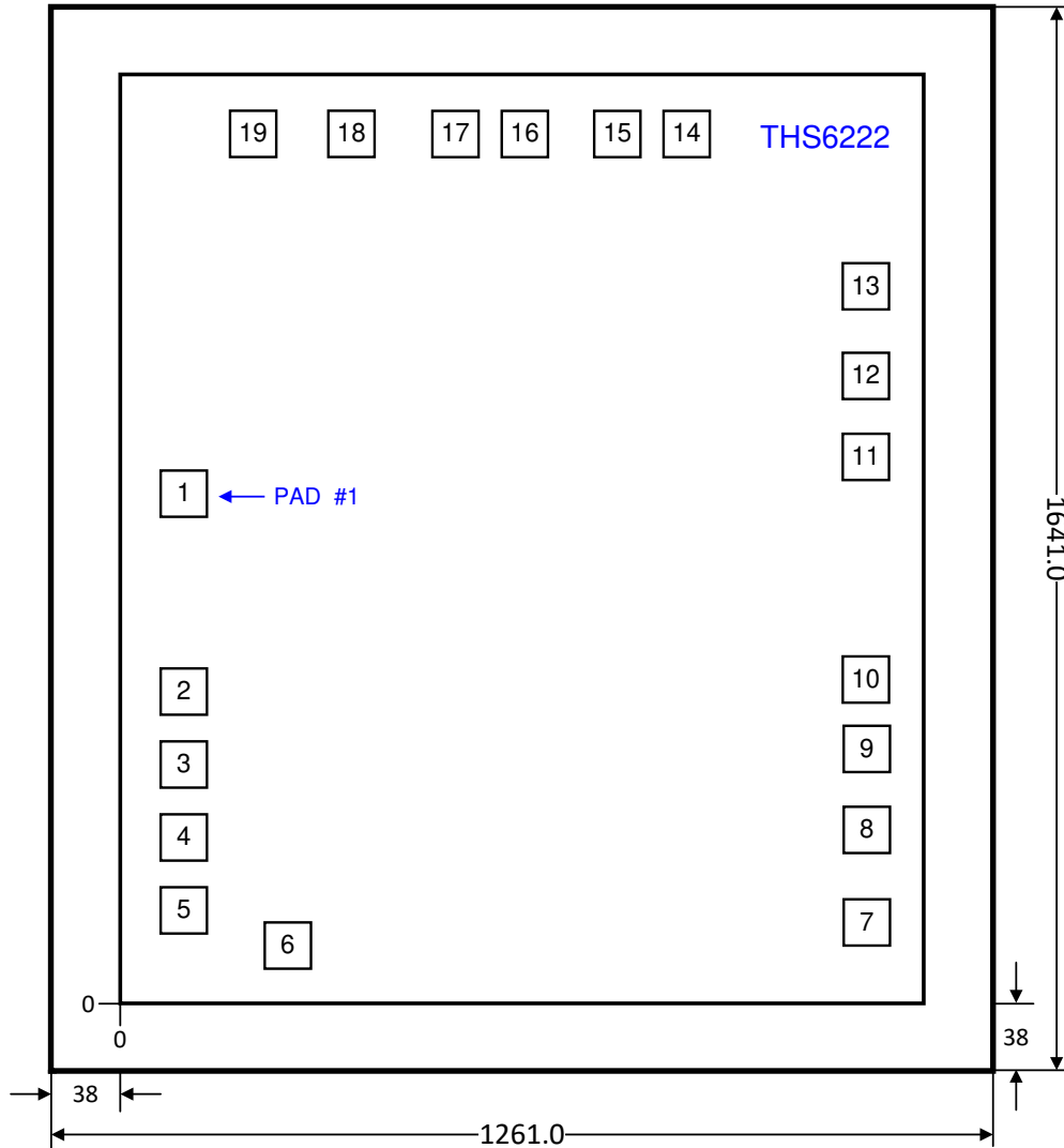
Figure 7-4. Die Dimensions
