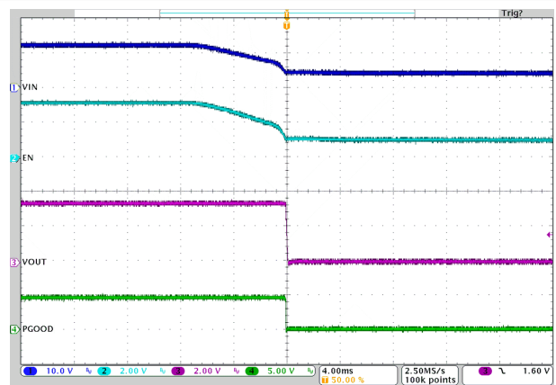
Figure 8-11. EN Shutdown
