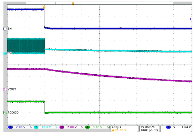
Figure 8-11. EN Shutdown
