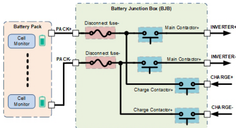
그림 1. 배전에서의 배터리 분리 퓨즈 및 고전압 릴레이
