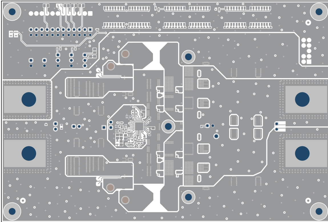
Figure 4-4. Top Layer
