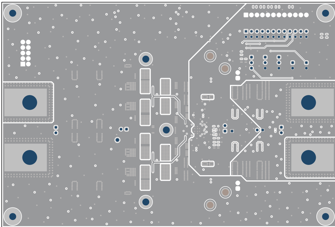
Figure 4-9. Bottom Layer
