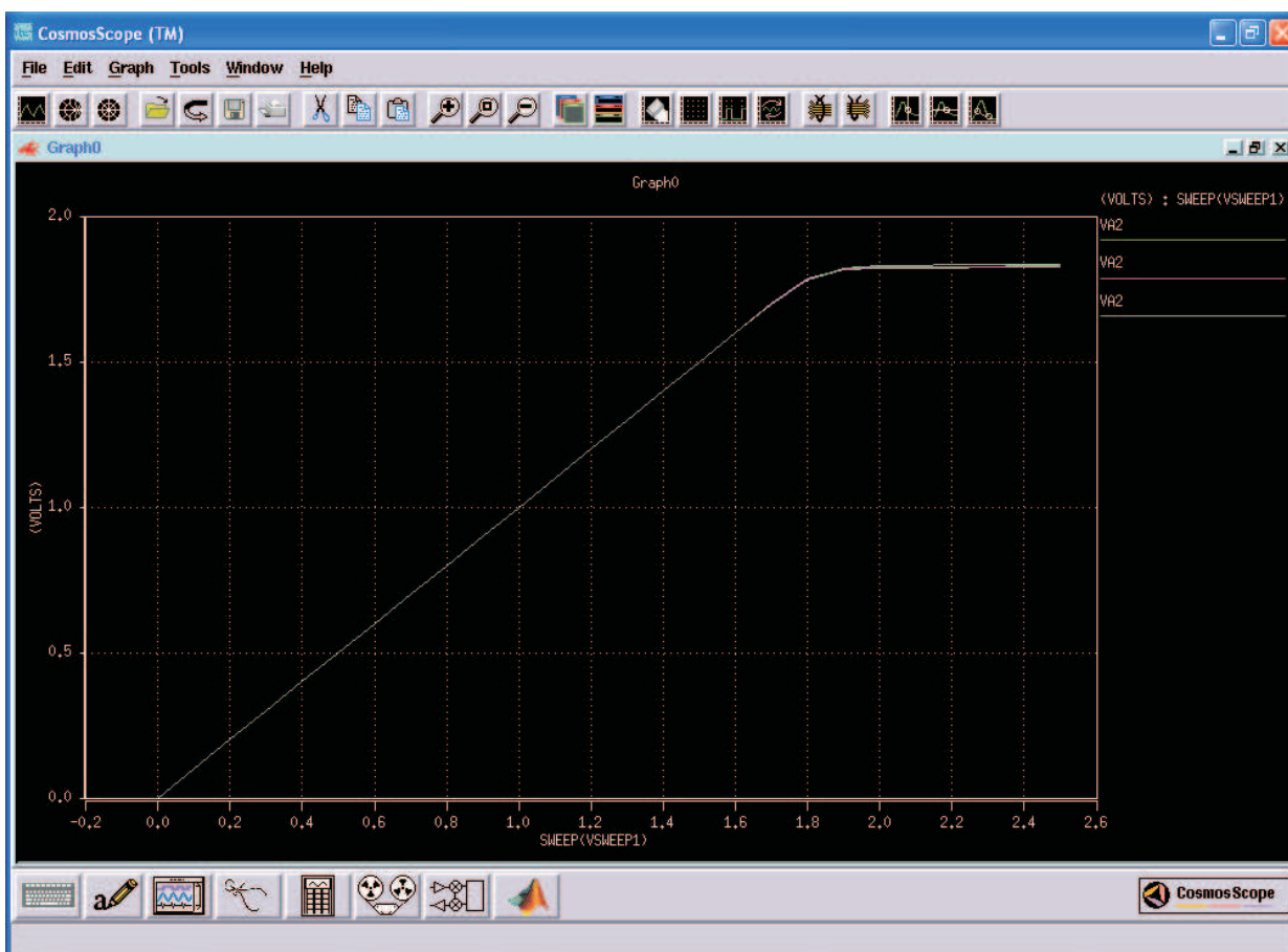
Figure A-2. VOUT vs VIN
