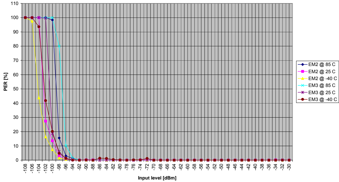
PER versus Input Level
