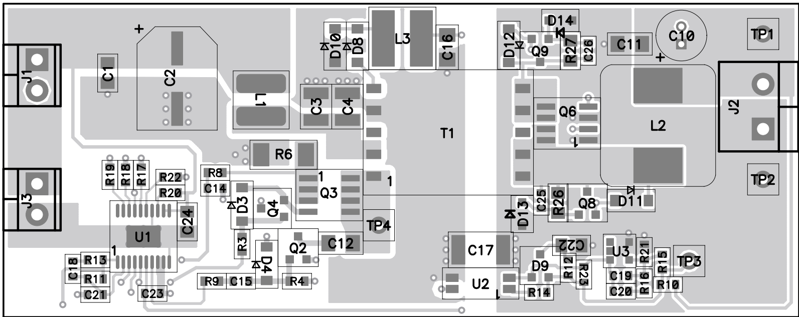
PMP4909 REV A LAYER 1-TOP
