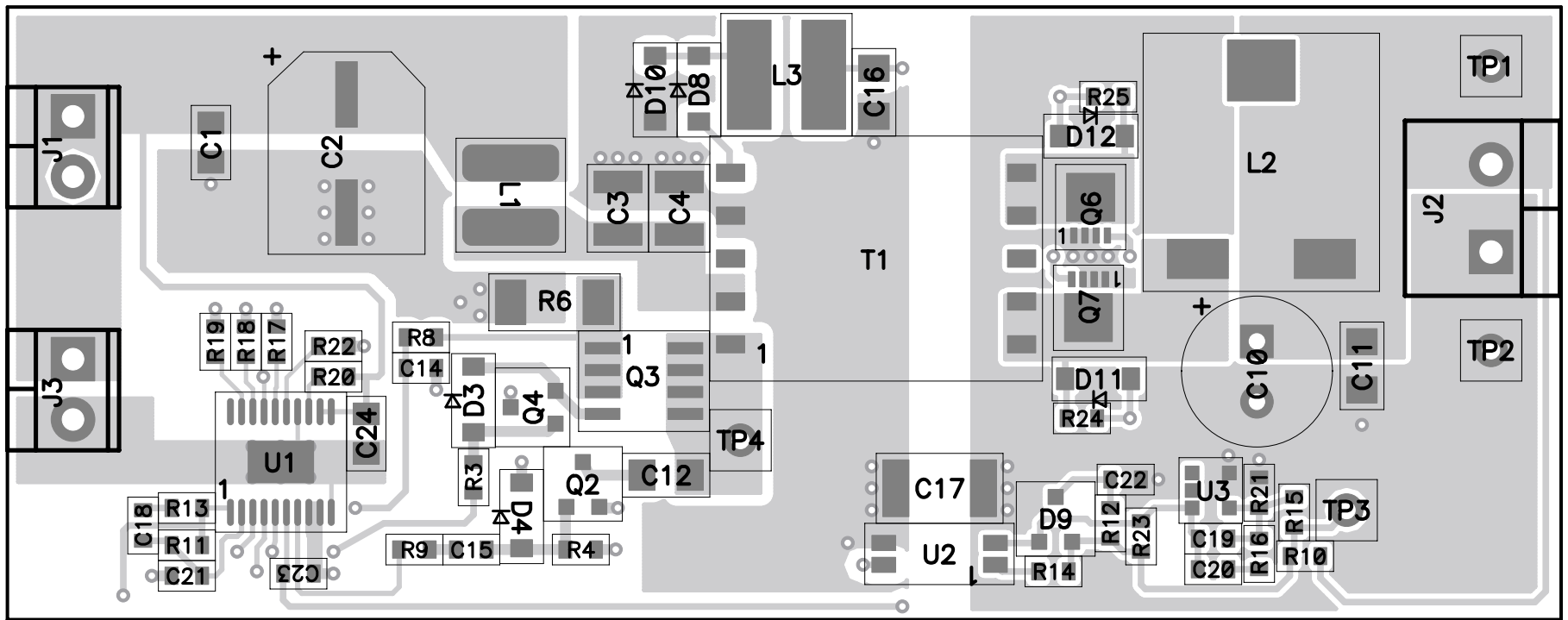
PMP4908 REV A LAYER 1-TOP
