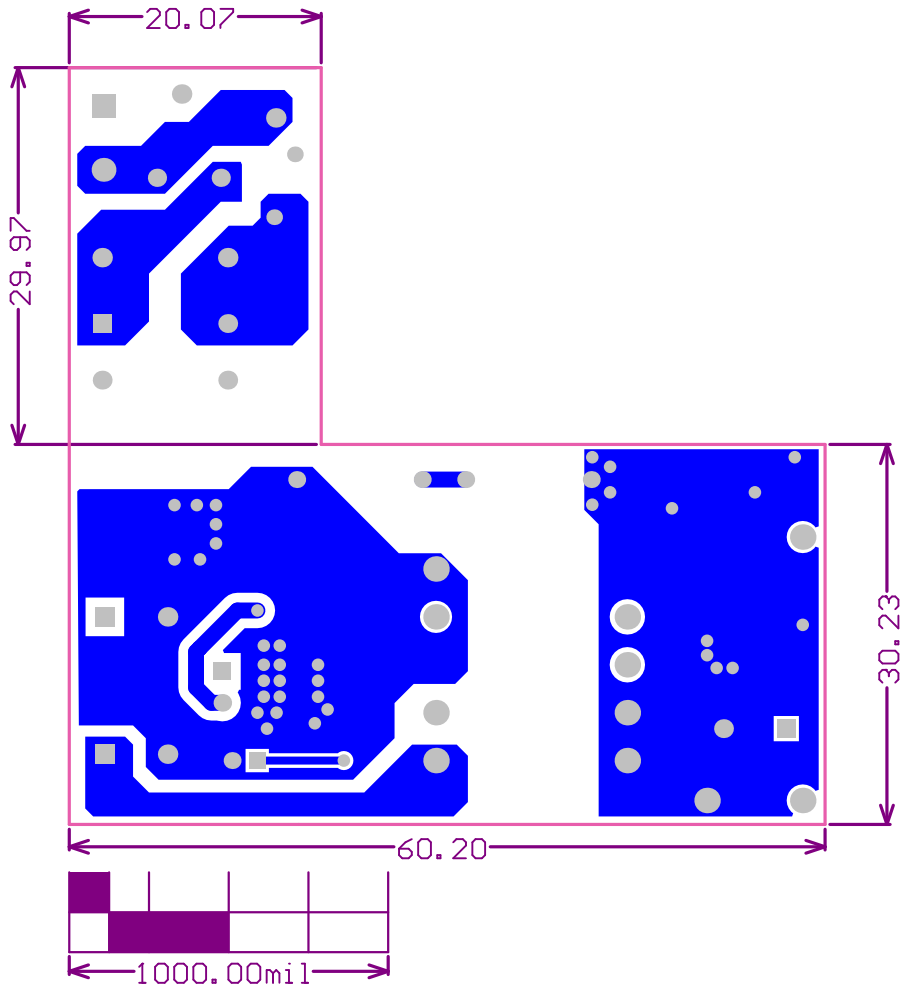
Bottom Layer M1 Board Outline
