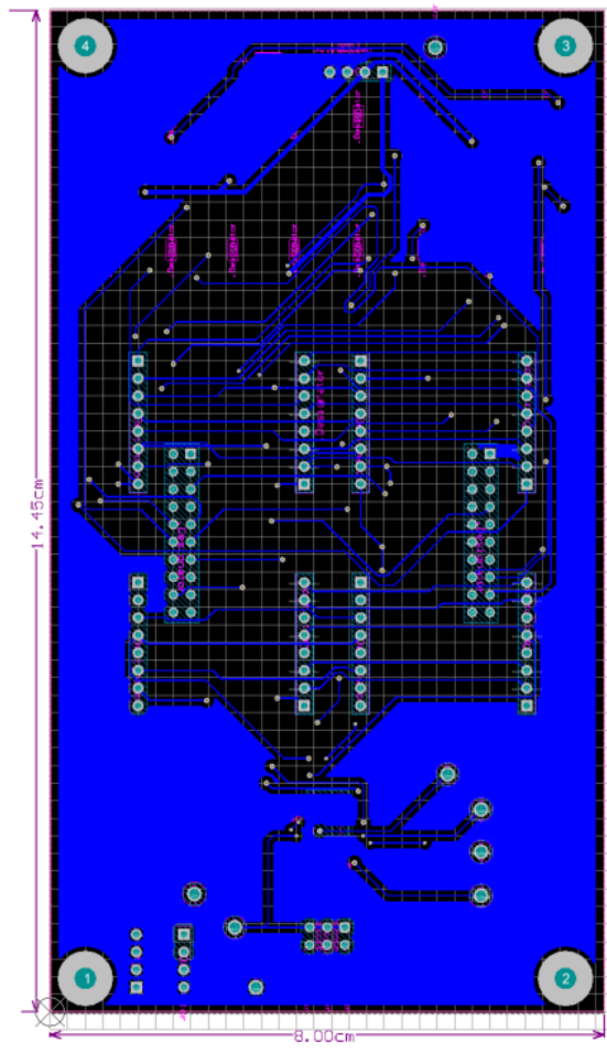
Bottom Layer
