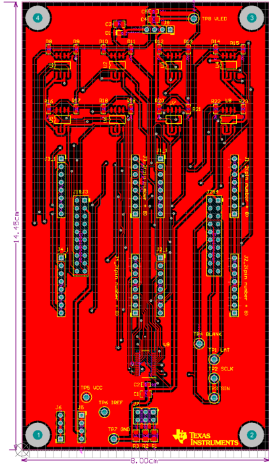
Top Layer
