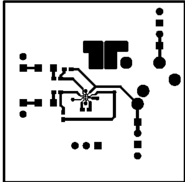
Figure 21. Top Layer
