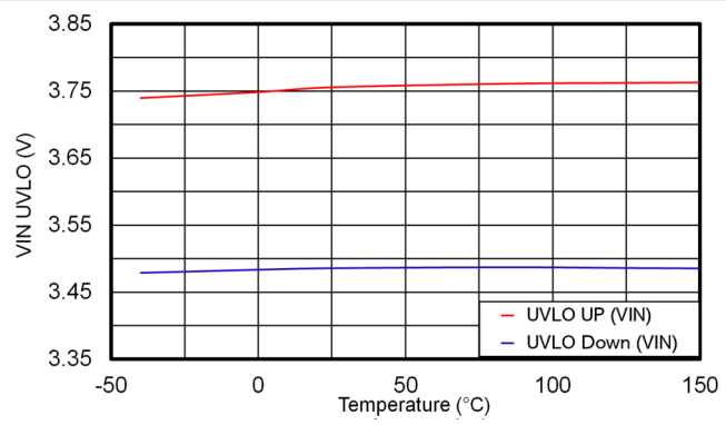
Figure 7-10. VIN UVLO
