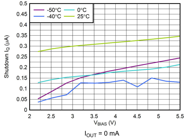
Figure 6-8. V_{\text{BIAS}} Shutdown I_{\text{Q}} vs V_{\text{BIAS}}
