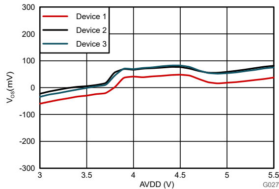
AMC0380D04-Q1
