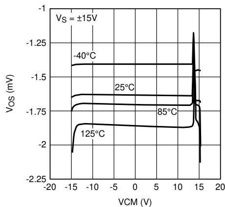
Figure 5-9. V_{OS} vs V_{CM} (Unit 1), Old Die
