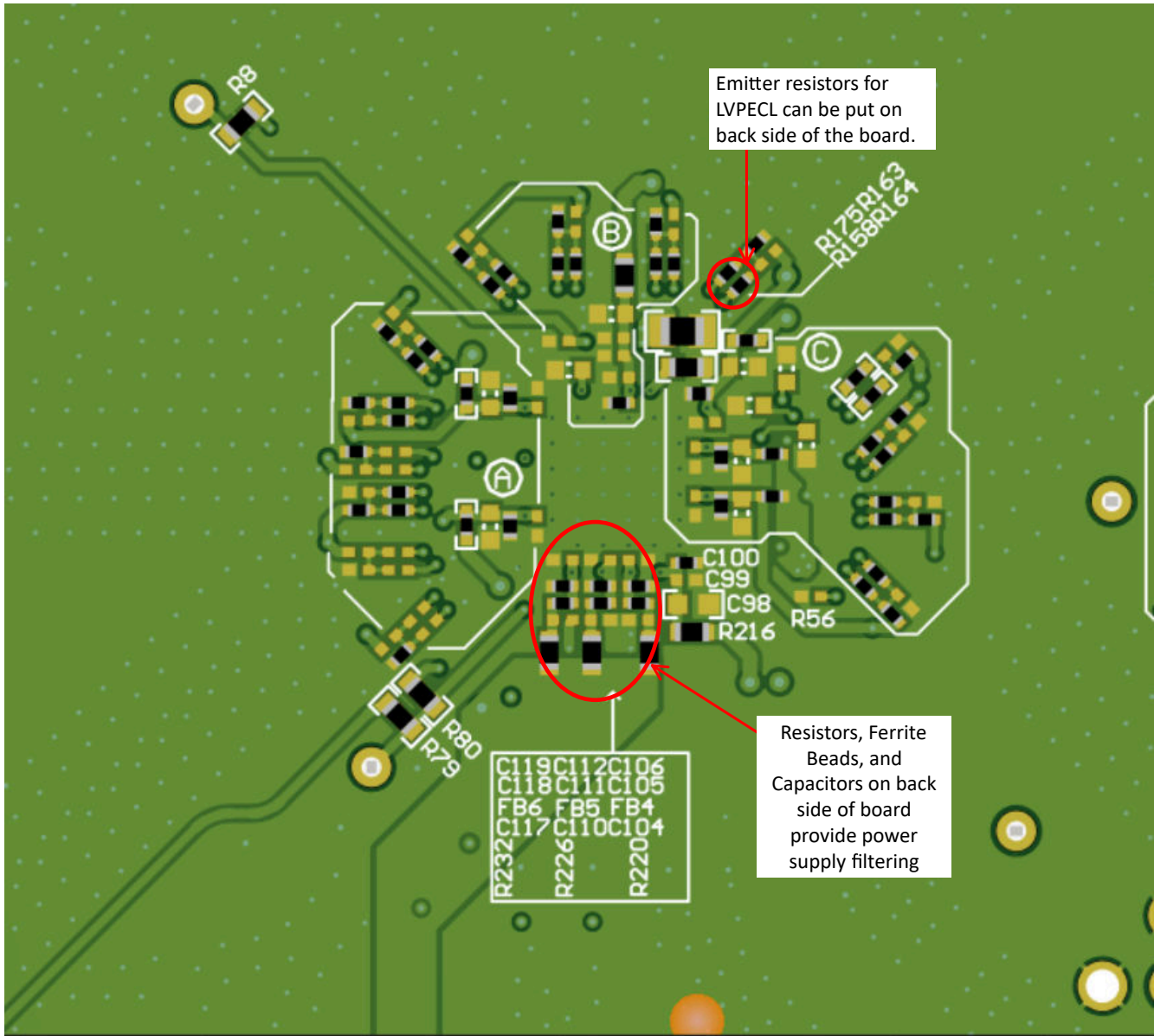
Figure 9-11. Bottom Layer
