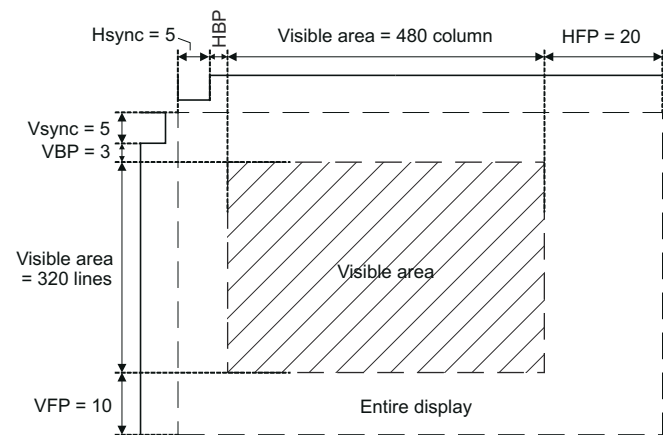
Figure 9-3. HVGA Display Parameters
