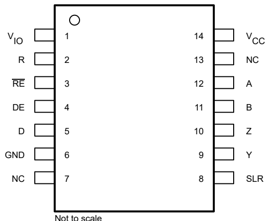
Figure 4-2. THVD2412V, THVD2452V 14-Pin SOIC Package (D) Top View
