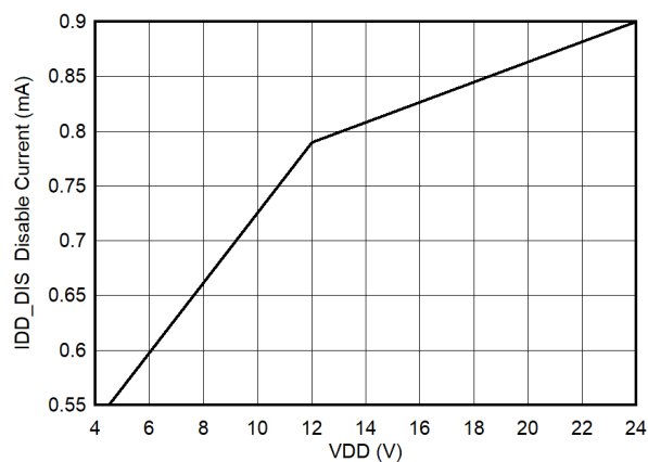
Figure 5-6. Disable Current (EN = 0 V)
