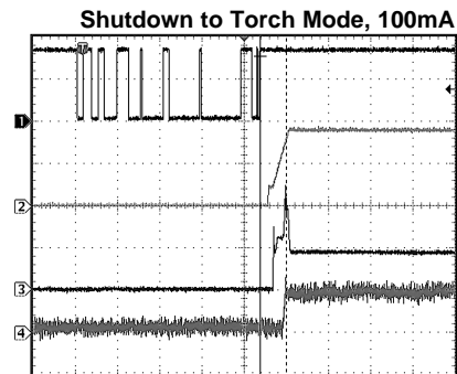
CH1: SDA; Scale: 2V/Div, DC Coupled CH2: V_{OUT} ; Scale: 2V/Div, DC Coupled CH3: I_{IN} ; Scale: 100mA/Div, DC Coupled CH4: I_{LED} ; Scale: 100mA/Div, DC Coupled Time scale: 400 \mu\text{s} /Div
