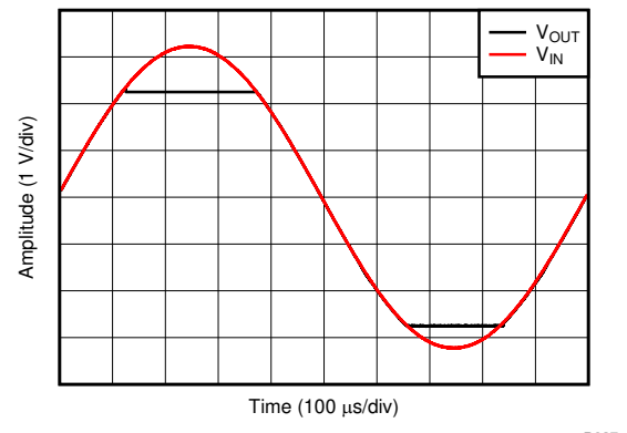
G = 1 V_{IN} = 6.5\text{ Vpp}
