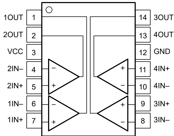
LM3302 Pinout
