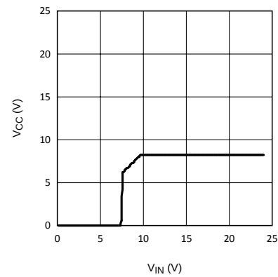
Figure 2. VIN UVLO
