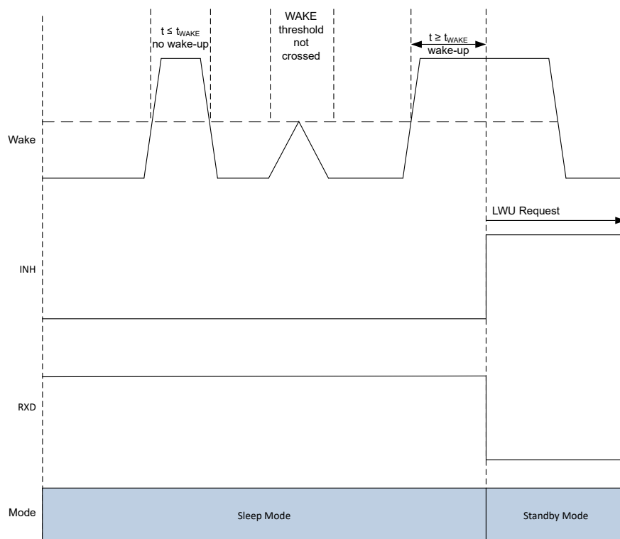
Figure 7-6. LWU Request Rising Edge
