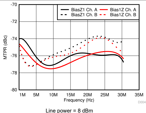
Figure 6-4. MTPR VDSL-30a Mode
