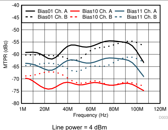
Figure 6-3. MTPR G.Fast 106-MHz Mode
