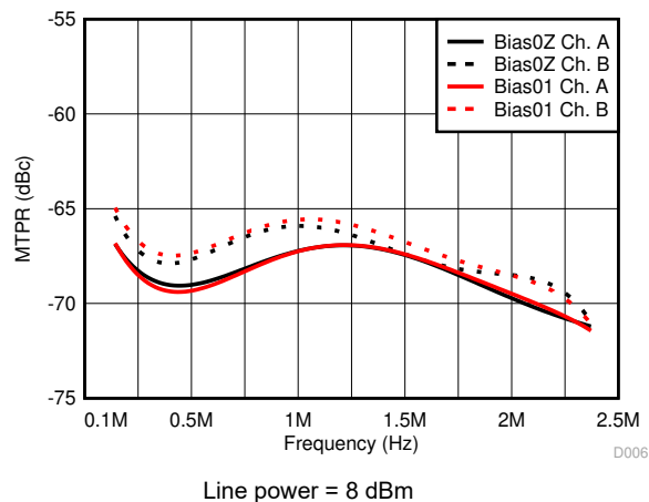
Figure 6-6. MTPR ADSL2+ Mode
