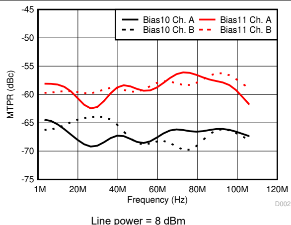
Figure 6-2. MTPR G.Fast 106-MHz Mode
