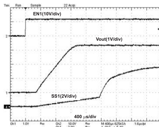
Figure 10. VO1=3.3V, SoftStart
