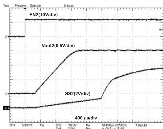
Figure 11. VO2=1.5V, SoftStart
