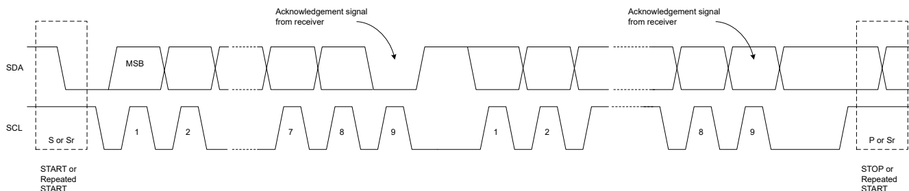
Figure 7-9. Byte Format
