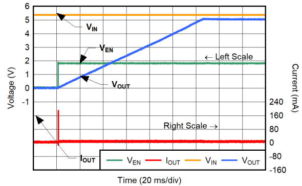
C_{NR/SS} = C_{IN} = 4.7\mu F , C_{OUT} = 22\mu F , V_{CP\_EN} = 0V , V_{BIAS} = 9V , V_{IN} = 5.5V , V_{OUT} = 5.2V
