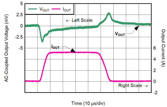
Time (10 \mu s/div ) C_{NR/SS} = C_{IN} = 4.7\mu F , C_{OUT} = 22\mu F , V_{CP\_EN} = 0V , V_{BIAS} = 11V , V_{IN} = 3.6V
