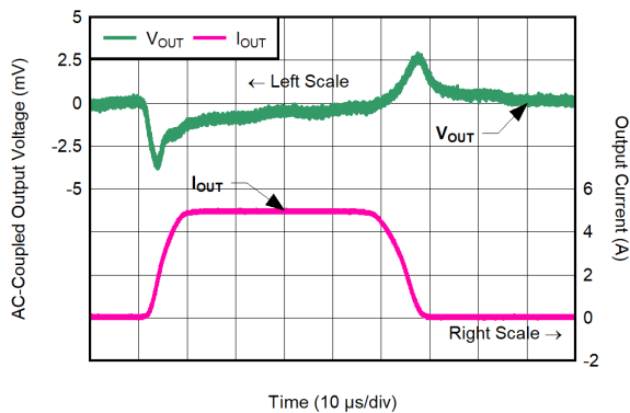
Time (10 \mu s/div ) C_{NR/SS} = C_{IN} = 4.7\mu F , C_{OUT} = 22\mu F , V_{CP\_EN} = 0V , V_{BIAS} = 11V , V_{IN} = 5.5V
