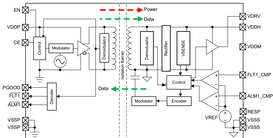
Figure 8-1. TPSI310x-Q1, TPSI310xL-Q1
