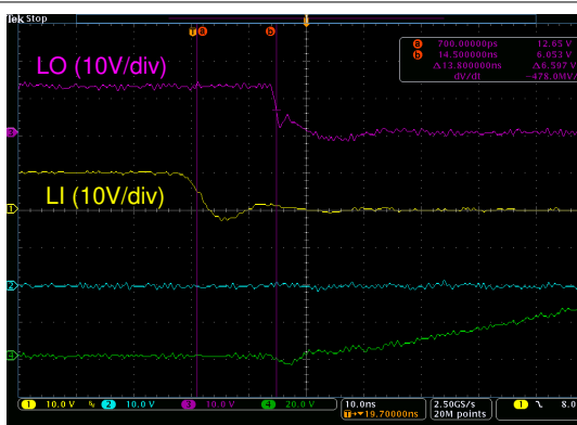
Figure 8-6. LO Fall Time
