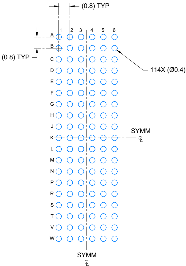
LAND PATTERN EXAMPLE SCALE: 6X
