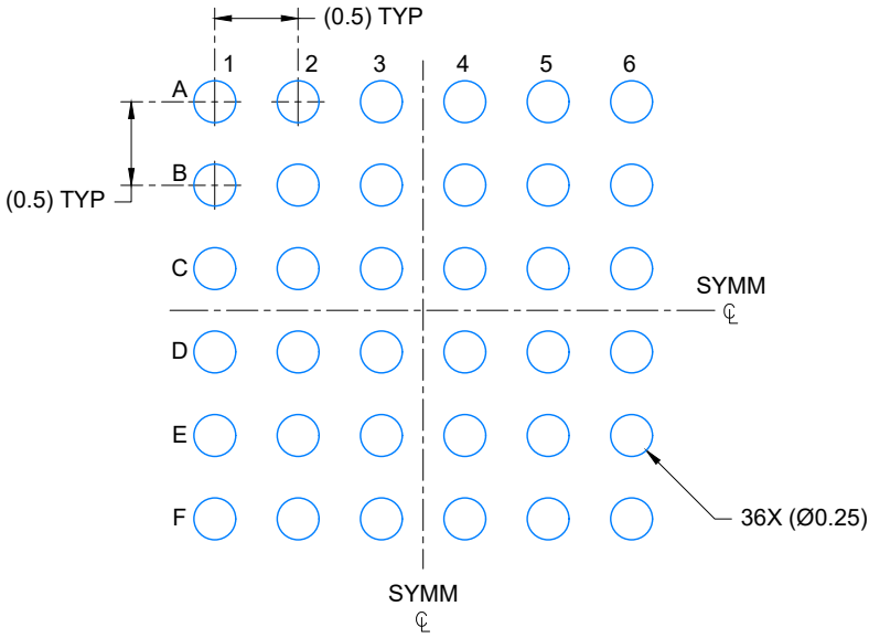
LAND PATTERN EXAMPLE SCALE: 20X
