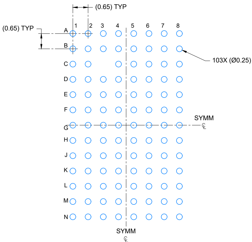
LAND PATTERN EXAMPLE SCALE: 10X
