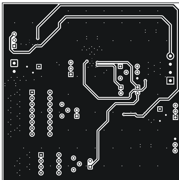
Figure 3-4. Bottom Layer
